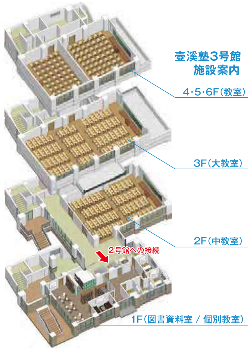
6階教室
